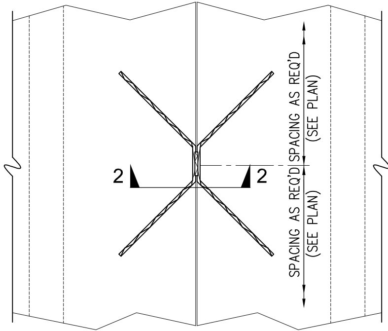
1 PLAN SCALE: 3/4" = 1'-0"
